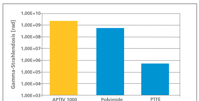
Abbildung 4: Strahlungsbeständigkeit
