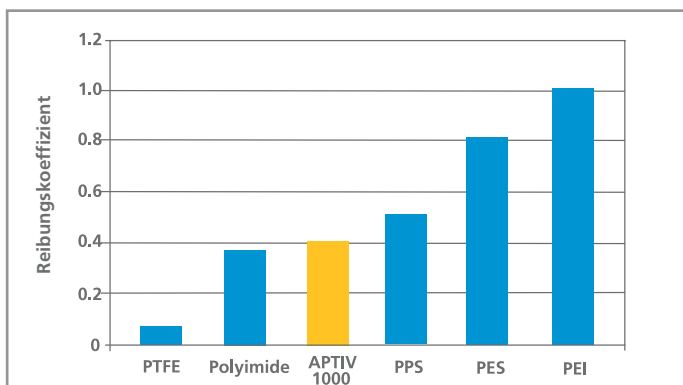
Abbildung 6: Dynamischer Reibungskoeffizient
