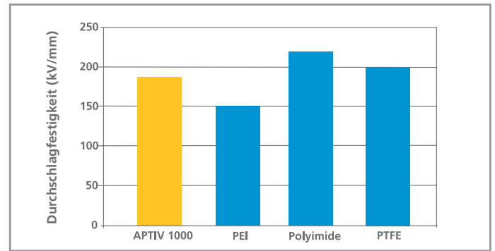
Abbildung 11: Durchschlagfestigkeit [50 µm Folie, 23 °C]
