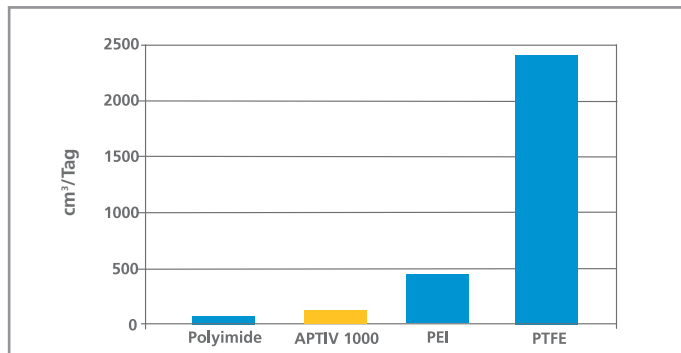
Abbildung 10: Sauerstoffpermeation bei 23 °C, 50 µm Folie, 0 % rel. Luftf.
