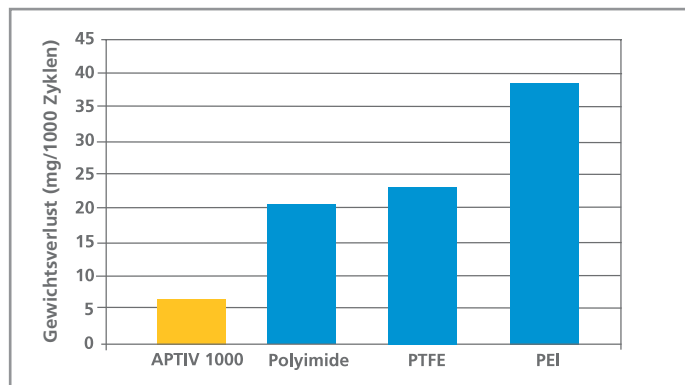
Abbildung 8: Abrieb nach Taber bei 23 °C
