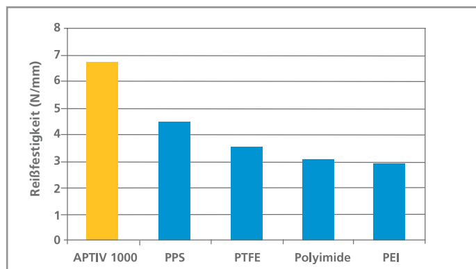
Abbildung 7: Reißfestigkeit bei 23 °C
