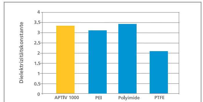
Abbildung 12: Dielektrizitätskonstante bei 23 °C
